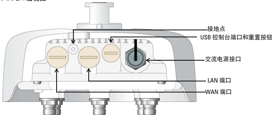
图 3 W-IAP274 后视图
