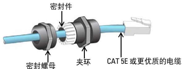
图 10 安装电缆密封套
