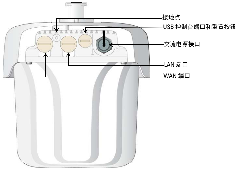
图 4 W-IAP275 后视图
